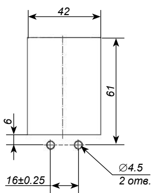
РПУ-2М102
