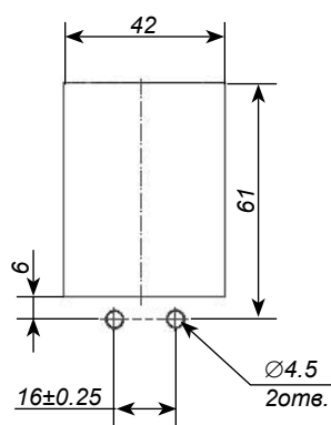
РПУ-2М202
